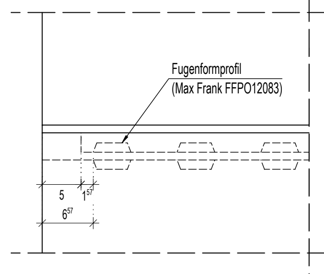
Ansicht Stoßfuge - Detail 1 M 1:5
