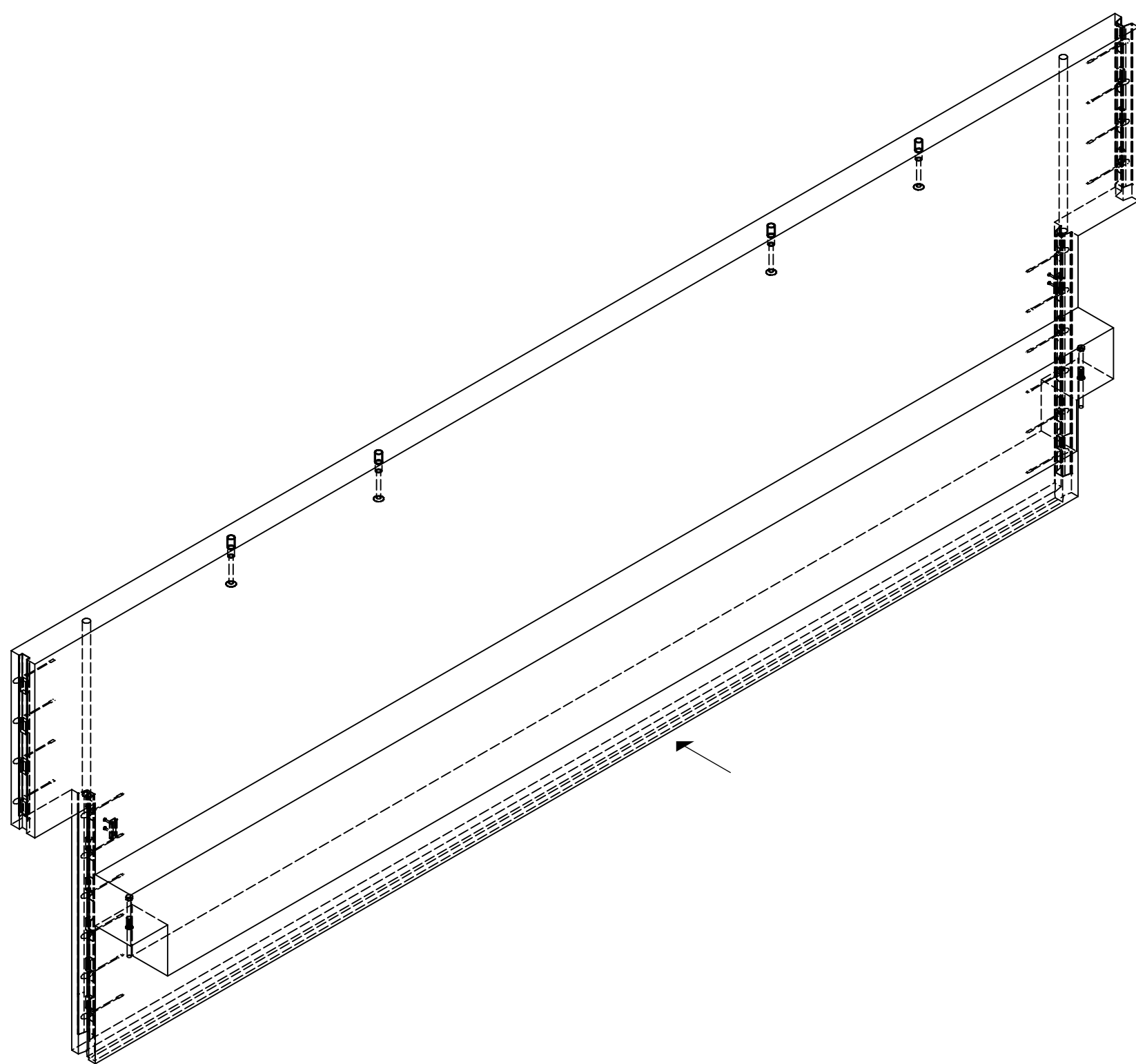
3D Perspektive M 1:25
