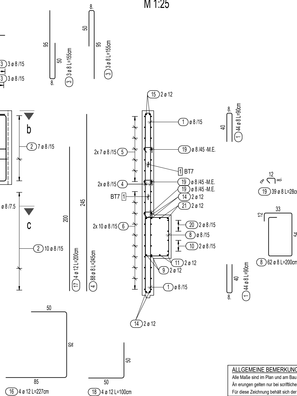
Schnitt a-a M 1:25
