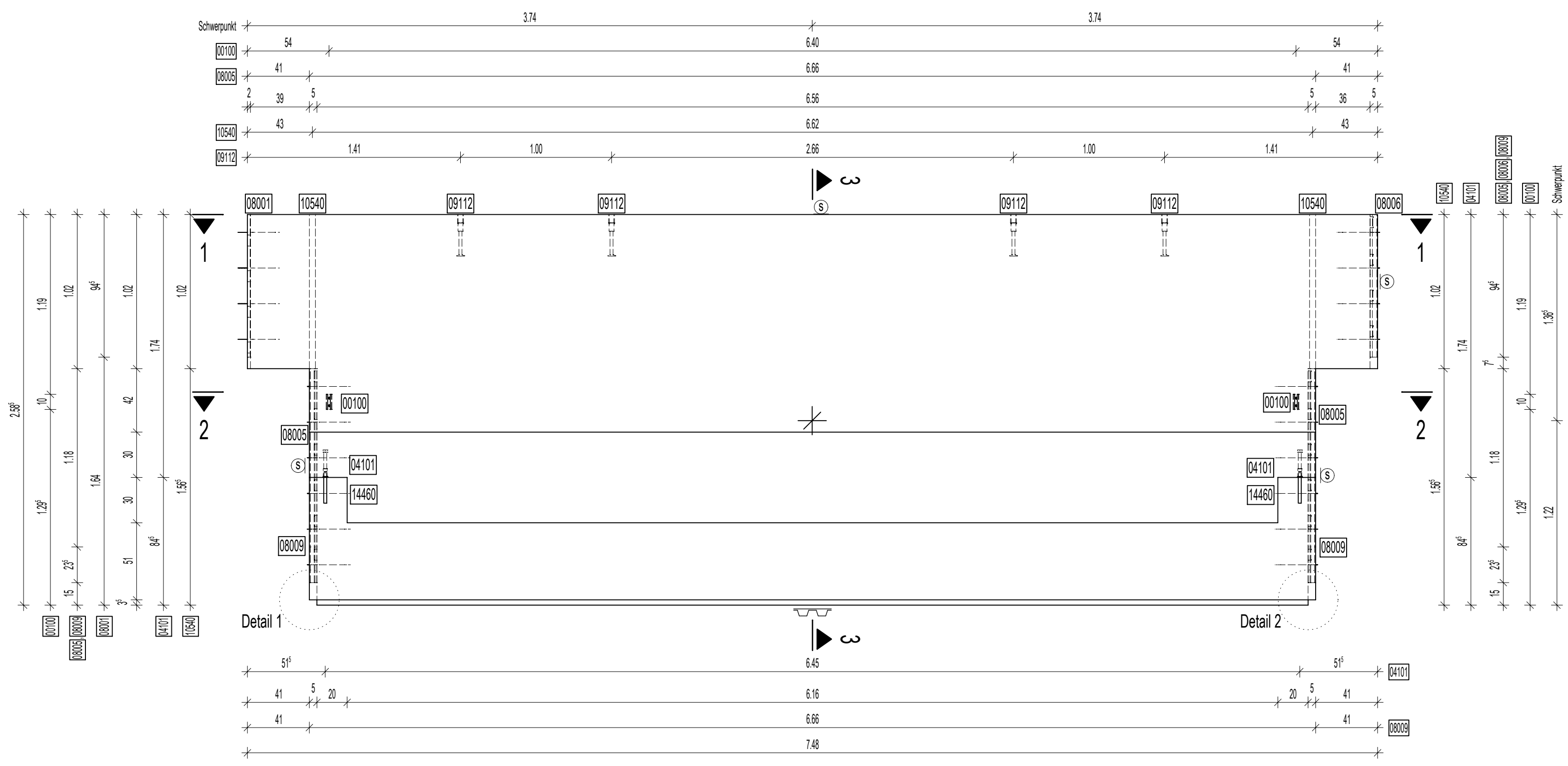
Draufsicht 1-1 M 1:25
