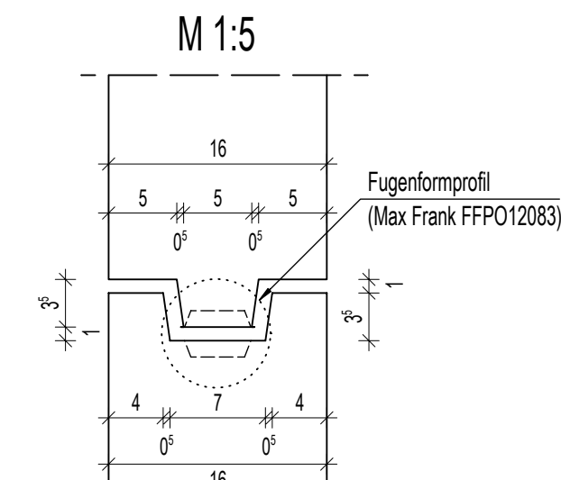
Detail Stoßfuge M 1:5
