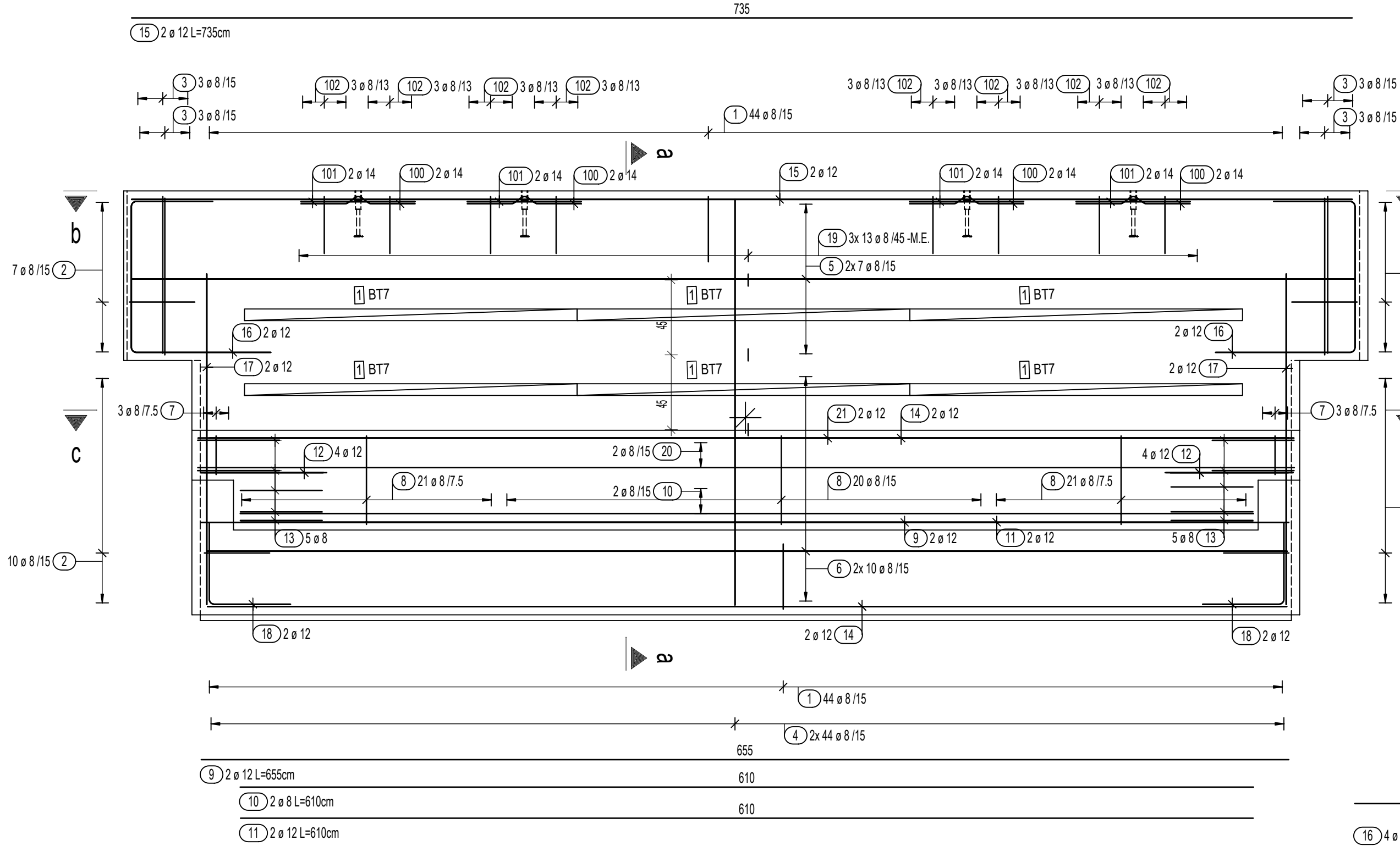
Bewehrung M 1:25
