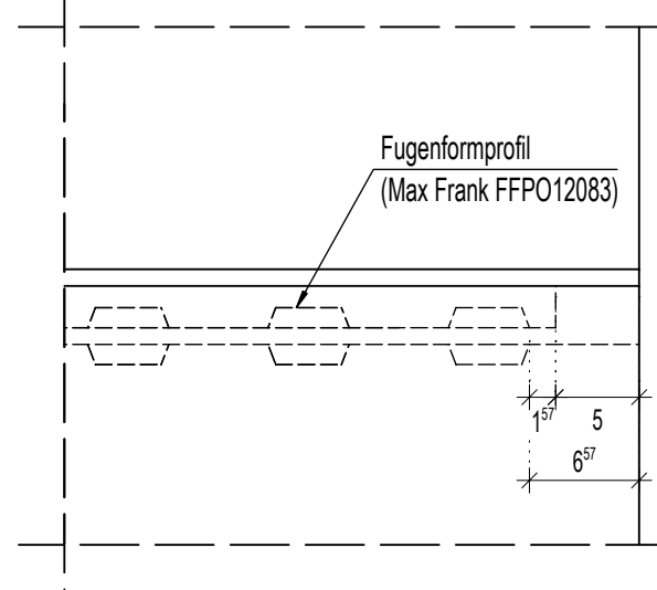
Detail Stoßfuge M 1:5
